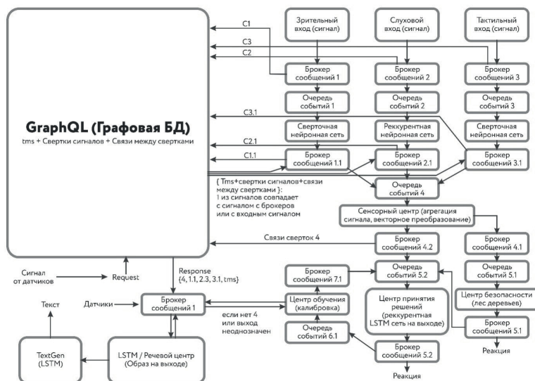
Рис. 3. Авторская архитектура искусственного интеллекта
