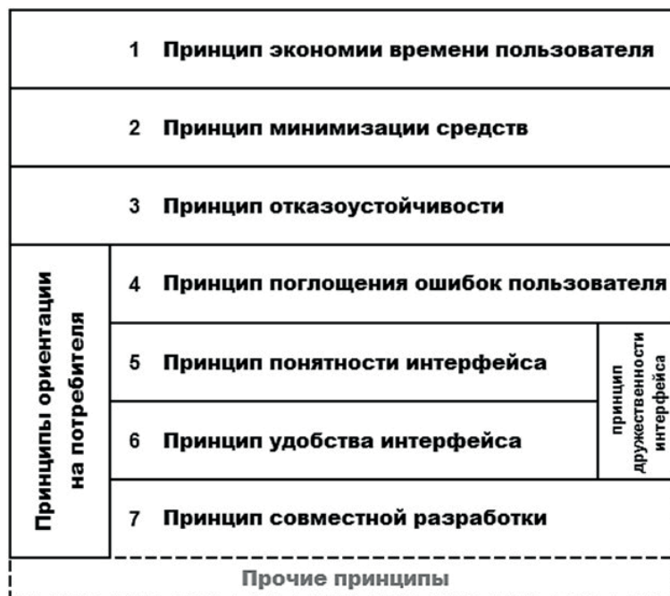
Рис. Иерархия принципов разработки компьютерных программ.
